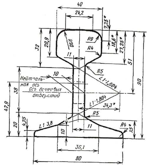
Рис. 2 Рельс Р18
