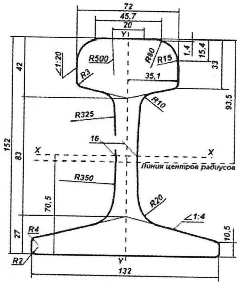
Рис.1 Рельс Р 50
